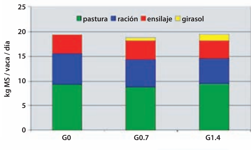
Figura 1- Consumo de pastura, ensilaje de trigo, ración comercial y semilla de girasol entera según nivel de suplementación.
